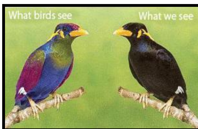
Obr. 2: Krkavcovití ptáci jsou ve skutečnosti pestrébarvní, lidské oko to jen není schopné rozlišit (zdroj: http://archives.evergreen.edu ).
