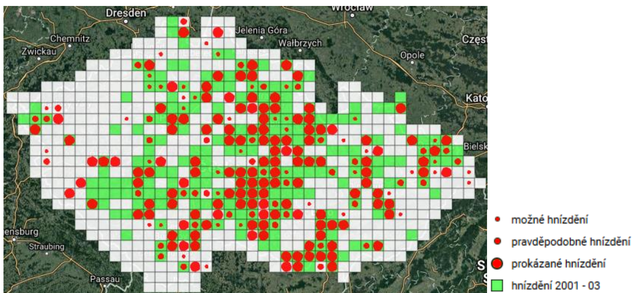
Obr. 1: Hnízdní rozšíření kavky obecné v ČR v letech 2001 – 2003 (zeleně) a průběžné výsledky z mapování v letech 2014 – 2017 (červeně), které ukazují na výjimečnost Vysočiny v rámci celé České republiky (zdroj: http://atlas.birds.cz ).
