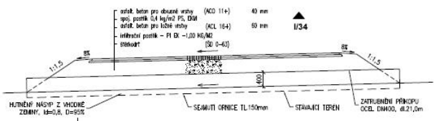
VZOROVÝ PŘÍČNÝ ŘEZ 1:50
