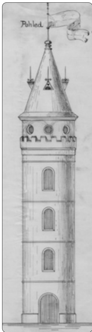
Výkres nerealizované rozhledny na Kalvárii (pohled, r. 1899)
