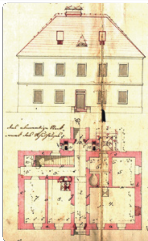
Škola ve Svatém Kříži mohla vypadat úplně jinak, kdyby na její stavbu byly peníze. Výřez z nerealizovaného plánu školní budovy z třicátých let 19. století.
